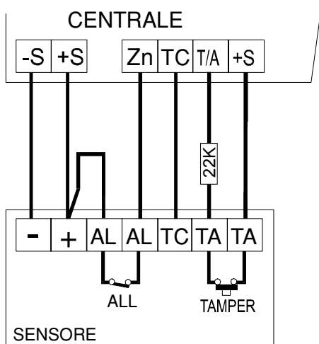
Esempio di collegamento di un sensore su zone programmate NC a positivo
