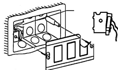
staffa supporto micro antimanomissione (MR03I) per l'utilizzo con scatole TICINO da incasso (503)
